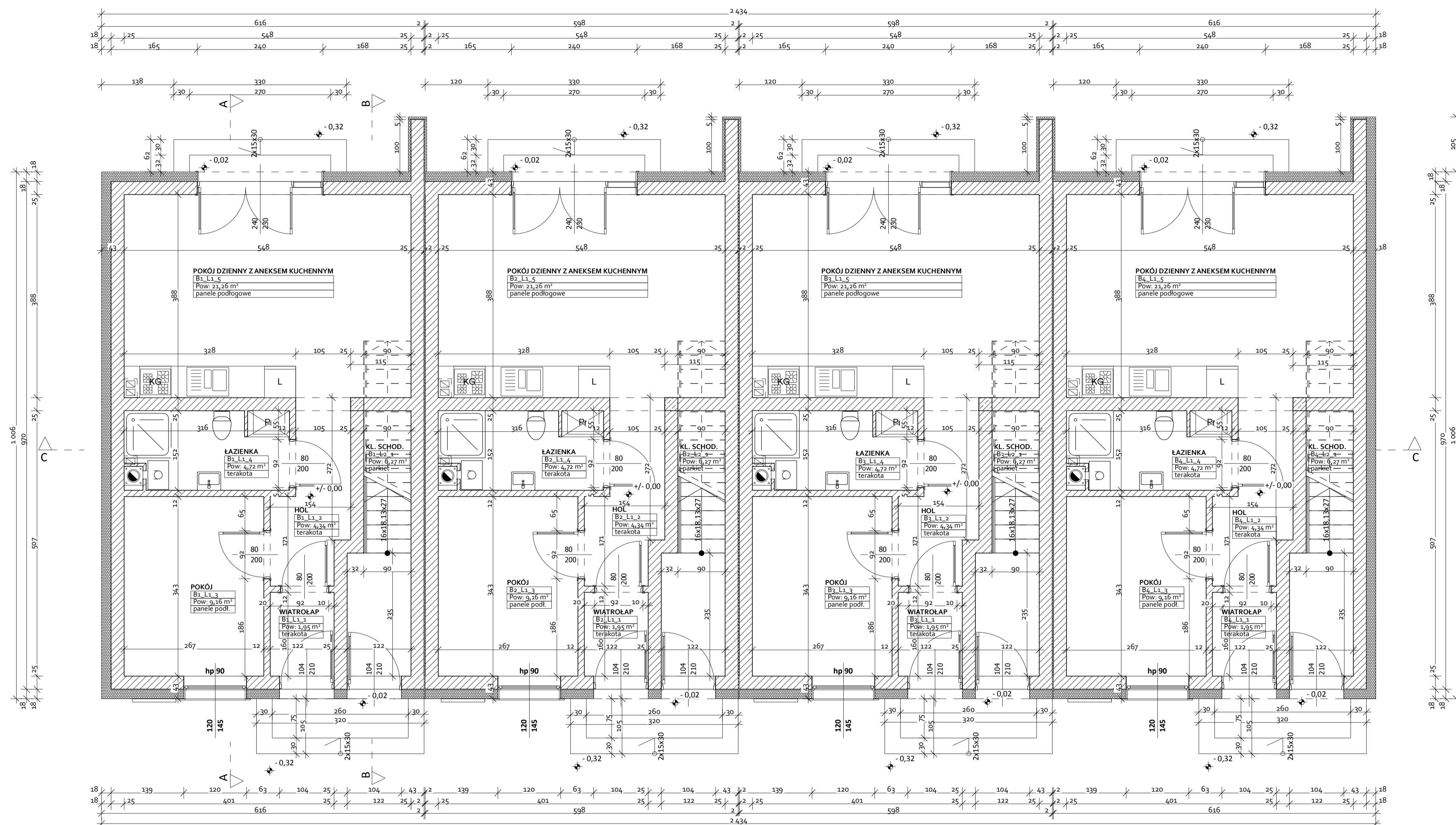
powierzchnia użytkowa obliczona wg PN-ISO 9836:1997 BUDYNEK MIESZKALNY "B1"
