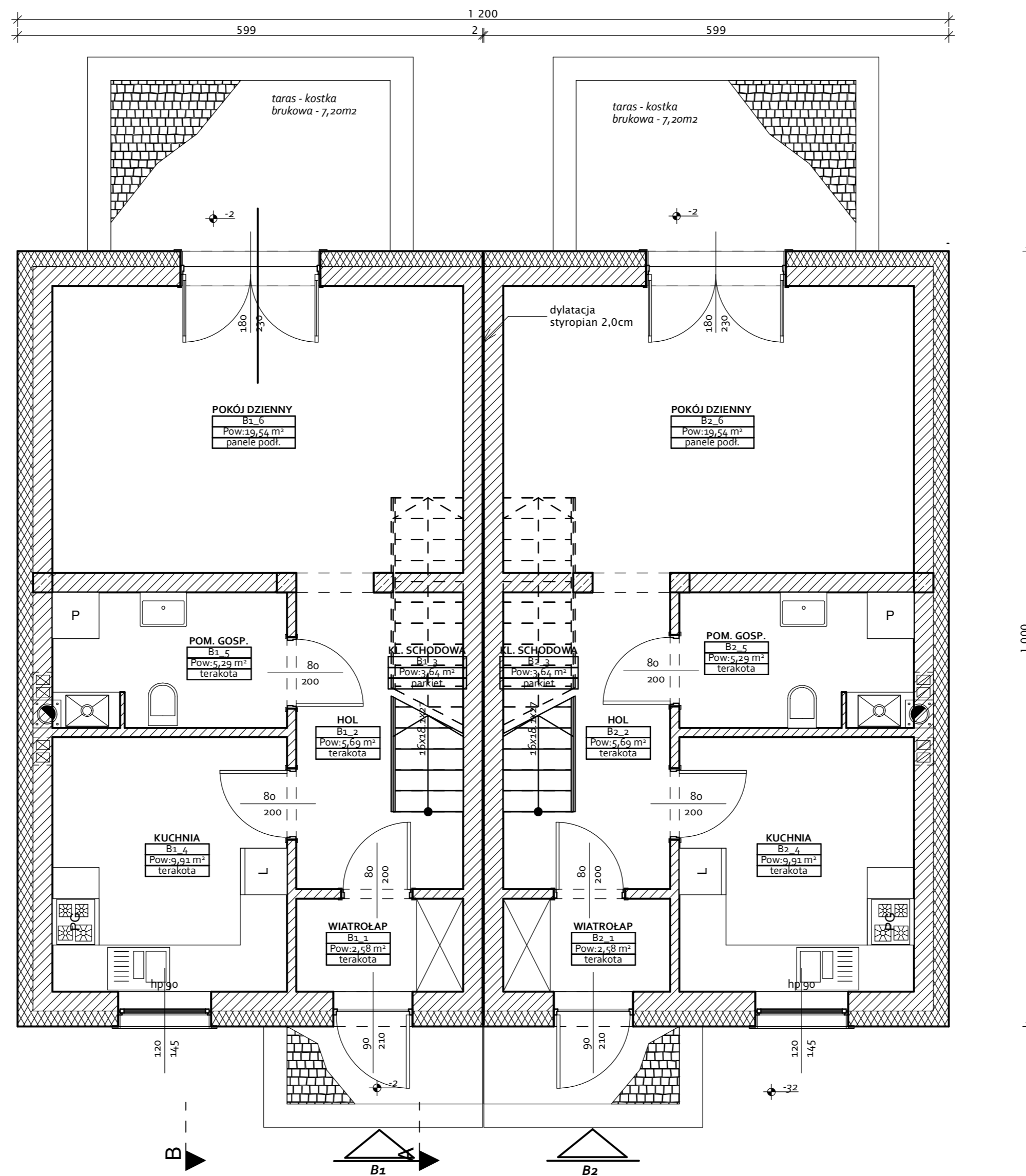
powierzchnia użytkowa obliczona wg PN-ISO 9836:1997 BUDYNEK MIESZKALNY "B1"
